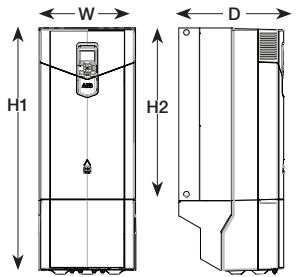
ACS880-01 R9
