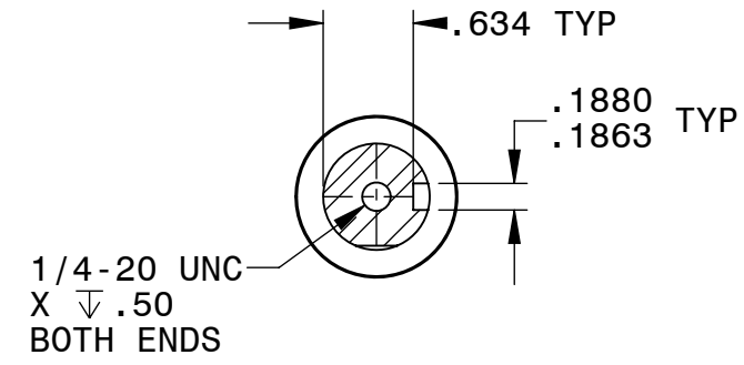
SECTION A-A SCALE 1 : 1.5
