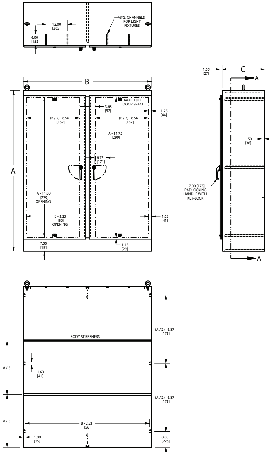
SECTION A-A
